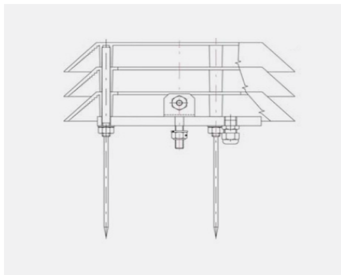
Иглы в нижней части служат для фиксации щита на поверхности земли
